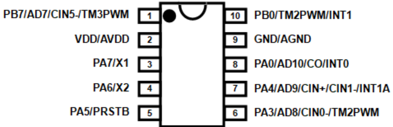
PMS171B-M10 (MSOP10-118mil)
