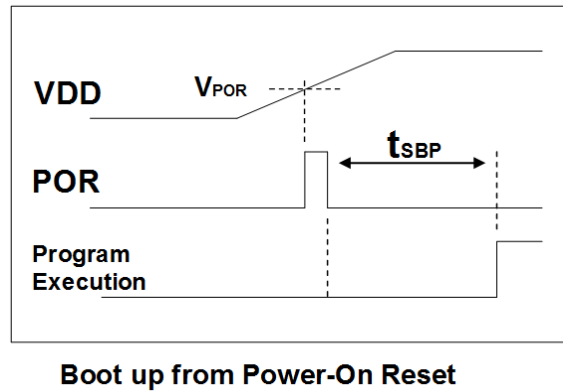
图 2：上电时序
